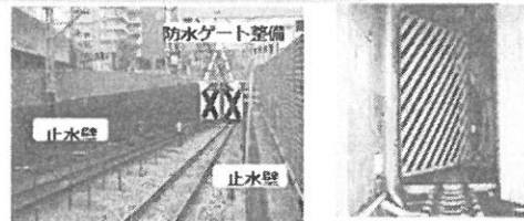
トンネル内防水ゲート
