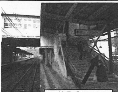
鉄骨ブレース
