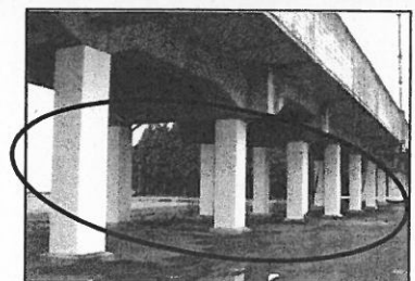
鋼板を巻く耐震補強により倒壊の被害なし
